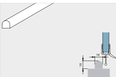
Bodemprofiel acryl transparant 10 mm / 1000 mm lengte
