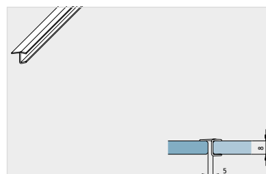
Aanslagprofiel 180° 2000 mm lengte
