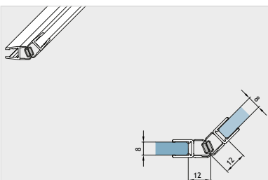
Magneet kunststof 135° 2200 mm lengte
