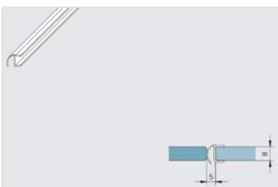
Middendichting 180° 2000 mm lengte, 5 mm
