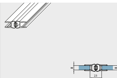
Magneet kunststof 180° 2200 mm lengte
