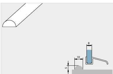
Bodemprofiel acryl transparant 5 mm / 1000 mm lengte
