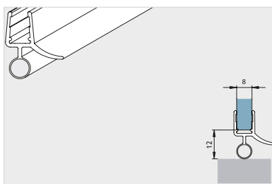
Lipdichting onderzijde lengte 1000 mm
