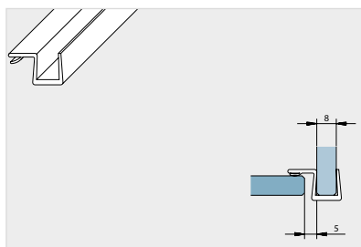
Aanslagprofiel 90° 2000 mm lengte
