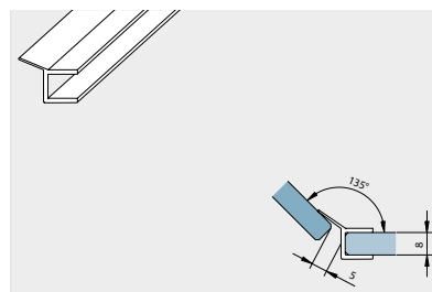
Middendichting 135° 2000 mm lengte
