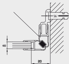
Magneet aansluitprofiel 2200 mm lengte
