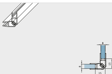
Magneet kunststof 2200 mm lengte
