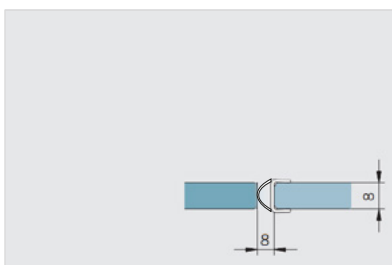
Middendichting 180° 2000 mm lengte, 8 mm
